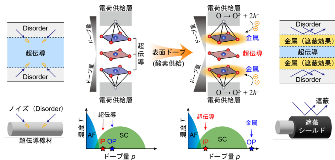
図 2：本研究で実現した「原子層レベルの金属シールド」と理想的な CuO 2 超伝導面。
