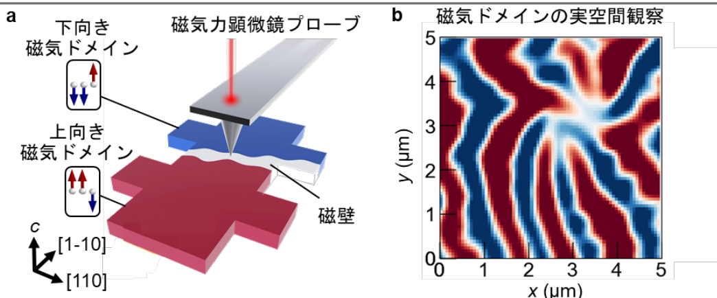
図2 磁気力顕微鏡を用いた磁気ドメインおよびその境界に現れる磁壁の実空間観察
