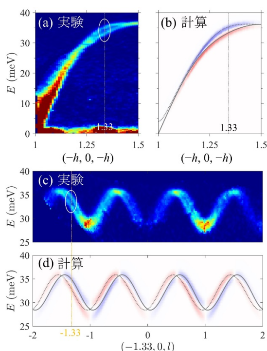
図 2 (a)&(c) MnTe の中性子スペクトル。それぞれ異なる運動量領域を示していますが、(a)の h = 1.33 と (c) の l = -1.33 は同じ運動量 (-1.33, 0, -1.33) となっています。この運動量では約 2 meV のマグノン分裂が観測されています。(b)&(d) 計算されたマグノンのカイラリティ。赤色と青色は各々異なるカイラリティを持つマグノンを示しています。灰色の実線および破線は計算されたマグノン分散を示しています。
