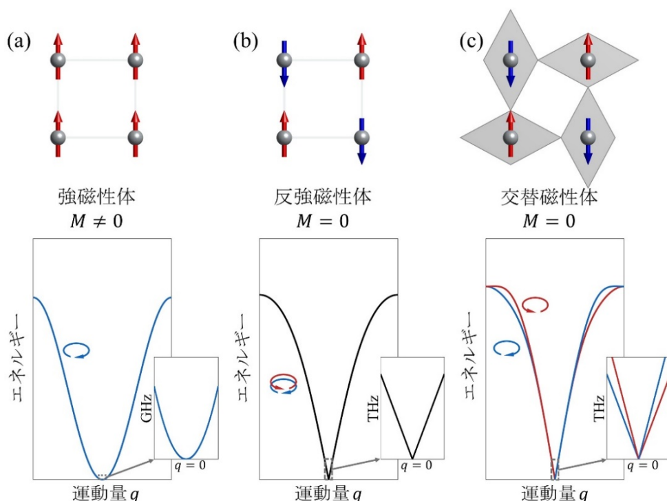
図1 (a) 強磁性体（第一の磁性体）、(b) 反強磁性体（第二の磁性体）、(c) 交替磁性体（第三の磁性体）におけるスピン構造（上）とマグノンのエネルギーと運動量の関係「分散関係」（下）の概略図。// は磁化を示します。分散関係に描かれている赤と青の矢印付き回転円は、各々反時計回り（右旋性）カイラリティ、時計回り（左旋性）カイラリティを表しています。
