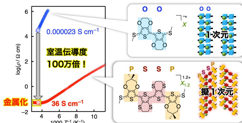
図3 新種のオリゴマー型有機伝導体の構造と電気伝導性
