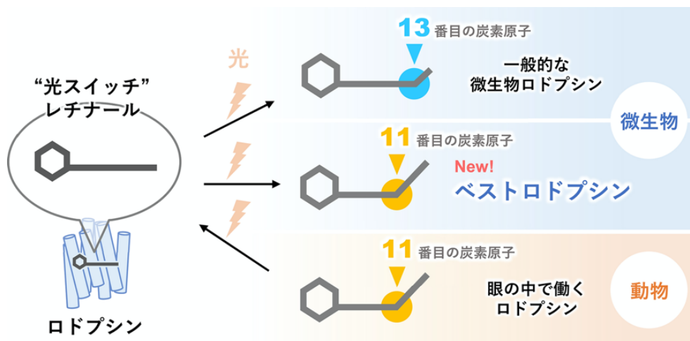
図 3 光によるレチナールの構造変化の比較。ベストロドプシンは微生物が持つロドプシンの仲間でありながら、動物のロドプシンと同じ箇所（11番目の炭素原子）でレチナールが折り曲がる。
