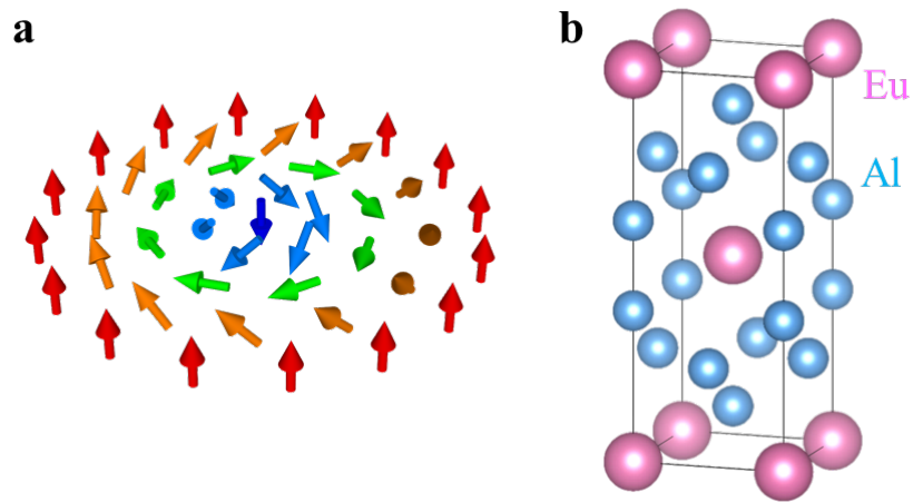
図1：(a) 一つの磁気スキルミオンの模式図。各矢印はユーロピウム (Eu) 原子それぞれの磁気モーメントの向きを示している。(b) \text{EuAl}_4 の結晶構造。
