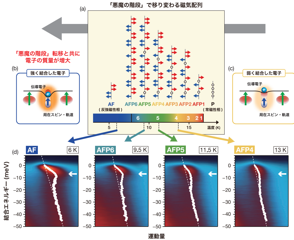
図2：(a) セリウム・アンチモンの「悪魔の階段」における磁気配列。(b, c) 「悪魔の階段」で変化する準粒子状態のイメージ。温度が低くなるにつれて、スピン・電子軌道との相互作用が段々と強くなり質量が増大しています。(d) 「悪魔の階段」に伴う準粒子の変化を観測したレーザー光電子分光の結果。「悪魔の階段」で起こる各磁気配列周期の変調に合わせて電子構造の折れ曲がり具合が大きく変化する様子が観測されました。
