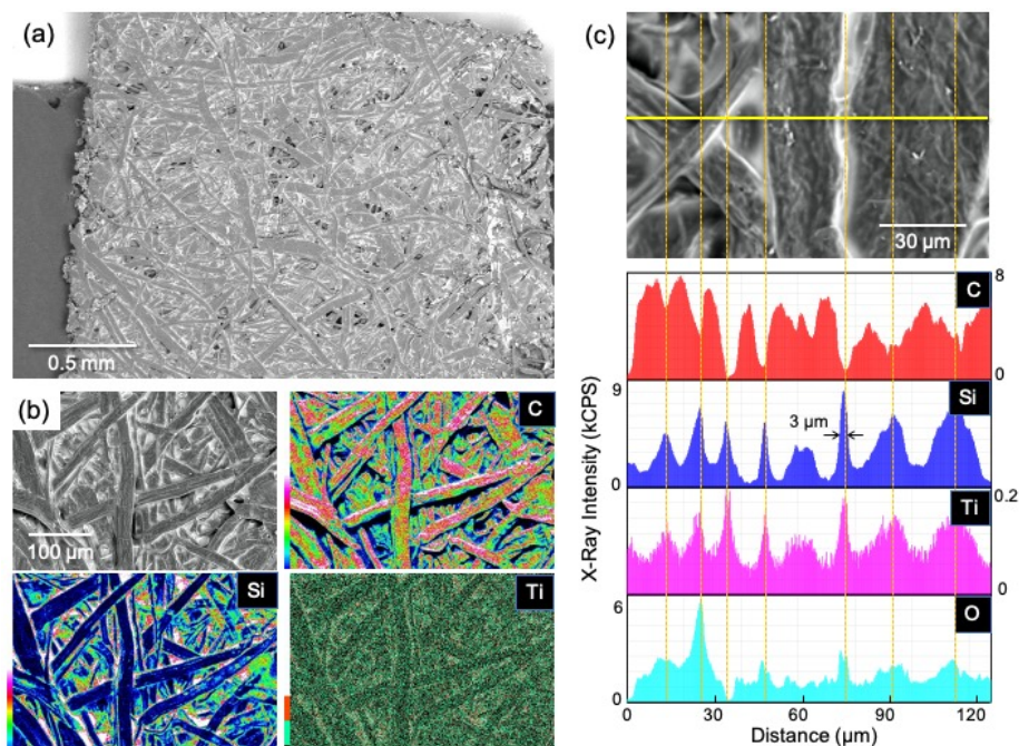
図1 コーティング紙の走査型電子顕微鏡（注5）像と元素マッピング。
