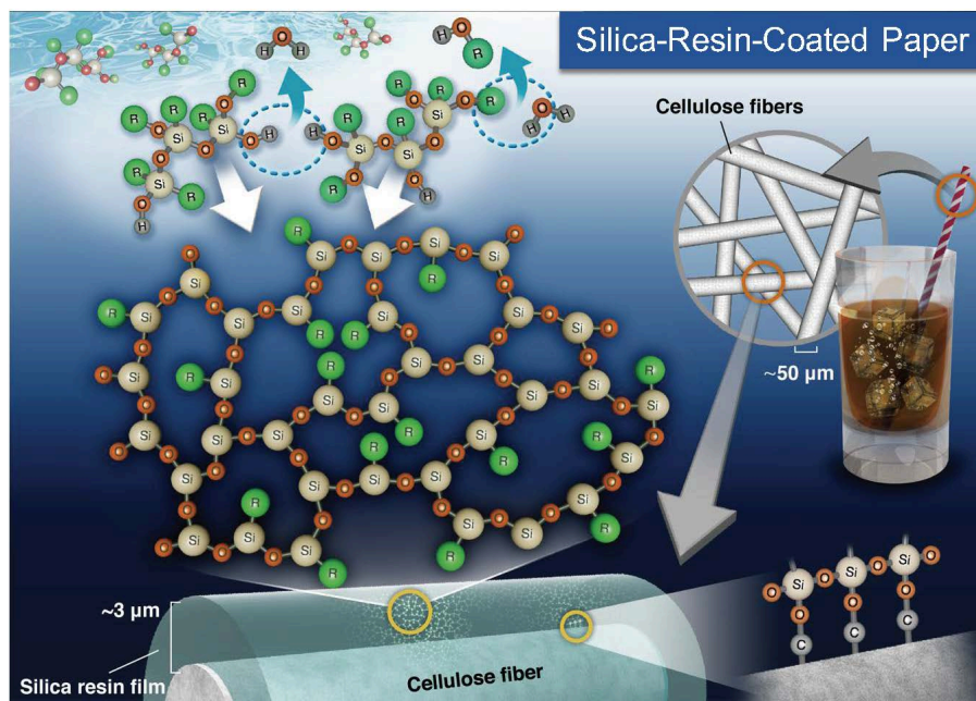
図2 超越コーティングにより、紙を構成するセルロースファイバー上にシリカ皮膜が形成される機構を説明する模式図。
