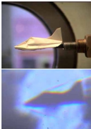
図 4 超越コーティングされた紙飛行機を用いて行われた空洞実験の様子[2]。下はマッハ 7 の風力で発生した衝撃波。
