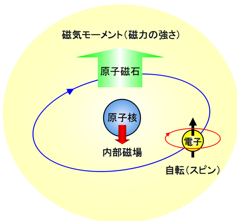
図1. 原子磁石の模式図。原子磁石の磁力（磁気モーメント）と原子核位置での内部磁場は、いずれも電子の自転（スピン）により互いに逆向きに生み出されます。本研究では、メスバウアー分光法 1) を用いて原子核位置での内部磁場を計測し、それにより原子磁石の磁性を評価しました。
