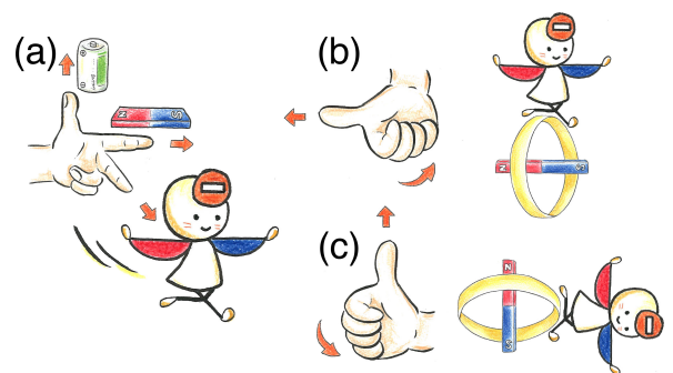
図1：電子密度の片寄りによる電子磁石の向きと、電子の軌道運動による電子磁石の向きの概念図。
