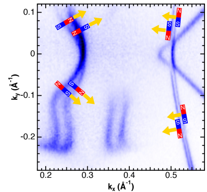
図2: シリコン表面上に作製したインジウム2層からなる原子層物質のフェルミ面。横軸と縦軸は電子のx方向とy方向の運動量(波数)です。いくつかの運動量における電子磁石の向きと電子が動く向き(黄色の矢印)。
