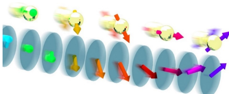
創発インダクタの概念図（上は電子とスピンを、下は電流駆動されたらせん磁気構造を表す）
