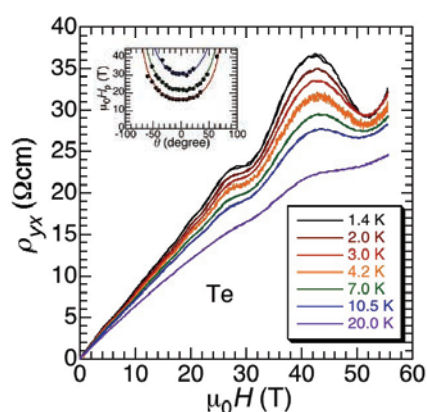
単結晶 Te のホール抵抗で観測した量子振動。(挿入図) ホール抵抗における微分ピークの磁場方位依存性。実線で示した二次元系で予想される振る舞いと一致は、この振動が二次元表面状態に起因することを示す。
