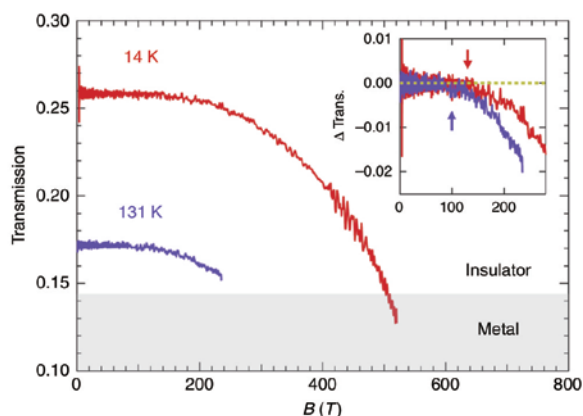
W を 6% ドープした \text{VO}_2 薄膜結晶の 1.977 \mu\text{m} の磁気透過測定結果。およそ 500 T で金属化による透過光強度の減少が観測されている。
