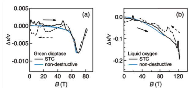
一巻きコイル法を用いた超強磁場音速測定の結果。(a) green diopside と (b) 液体酸素の音速の磁場依存性。
