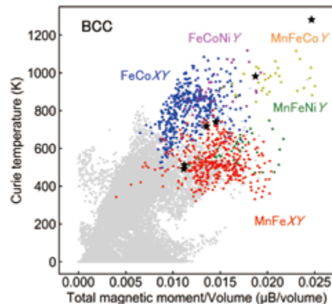
AkaiKKR コードを利用した 4 元磁性高エントロピー合金のハイスループット自動計算。Automatic high throughput screening of quaternary magnetic high entropy alloys by AkaiKKR code.
