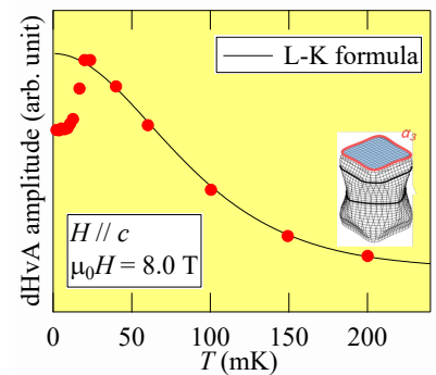
H. Shishido et al., Phys. Rev. Lett. (2018)
