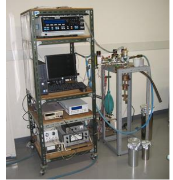
誘電率測定装置(柏)
