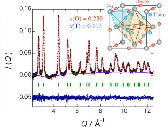
Pdナノ粒子の中性子回折
