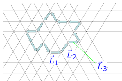
左図：三角格子上の量子ブラウン運動（摩擦力を受けながら量子力学的に運動する粒子）を表すダイアグラム。長距離におけるふるまいは、2成分自由ボソン場の共形不変な境界条件や、3本の量子細線の接合に対応する。 C. Chamon, M. Oshikawa, and I. Affleck, Phys. Rev. Lett. 91 , 206403 (2003); J. Stat. Mech. 0602 , P008 (2006).
