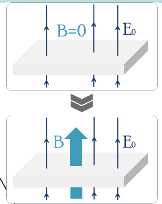
上図：アクシオン場の不安定性から導かれた、強電場下での自発的な磁場生成。 H. Ooguri and M. Oshikawa, Phys. Rev. Lett. 108 , 161803 (2012).
