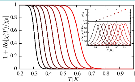
左図：理論的に予言された、さまざまな観測周波数についての超流動密度の温度変化。観測周波数が低くなるほど超流動「転移温度」が低下する。
