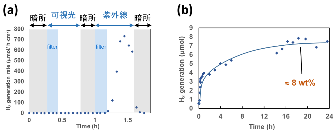
図3 (a)ホウ化水素シートからの水素放出特性(照射光の波長依存性。filter と記載されている領域は波長 490nm 以下の光をカットするフィルターを挿入) (b)紫外線照射時の水素生成能力
