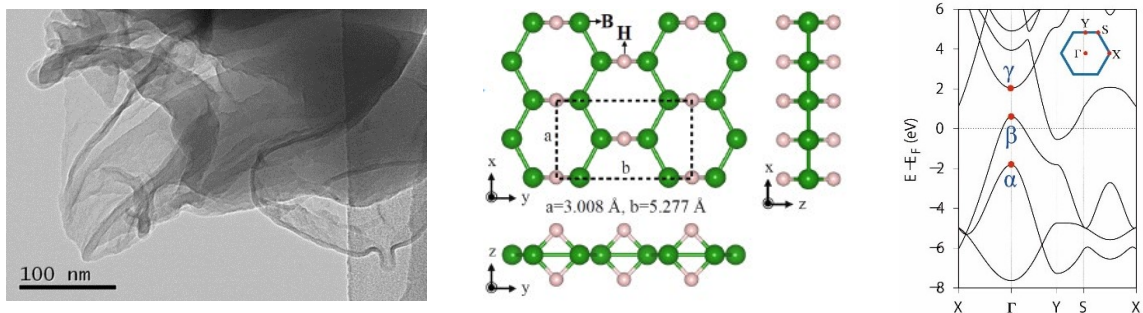
図2 ホウ化水素シートの透過型電子顕微鏡写真(a)、結晶構造(b)、電子構造(c)
