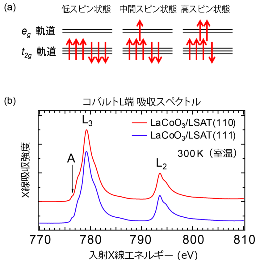
図 1 (a) : コバルトイオンのスピン状態の概略図。 e_g 軌道の電子の数によって低スピン状態 (0 個)、中間スピン状態 (1 個)、高スピン状態 (2 個) に区別される。(b) : コバルト L 端における吸収スペクトル。歪みの異なる 2 種類の薄膜のスペクトル形状に明確な違いは見られない。A の矢印は共鳴軟 X 線非弾性散乱に用いた入射 X 線のエネルギーを示している。
