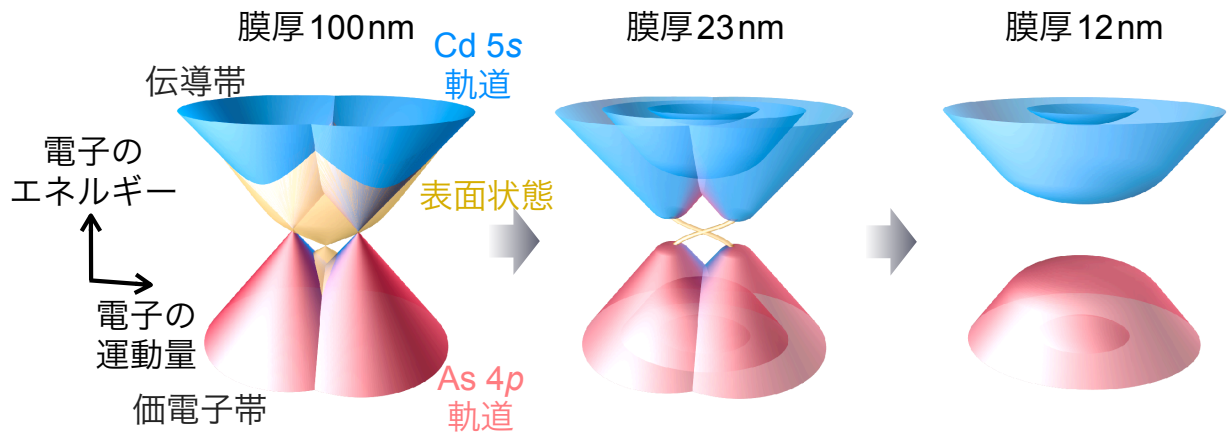
図1. \text{Cd}_3\text{As}_2 の電子構造と次元性の変化によるトポロジカル相転移の例
