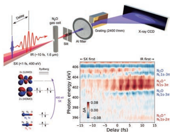
アト秒軟X線パルスを用いたN 2 O分子の過渡吸収分光と、内殻励起に関するエネルギー準位、観測されたサブサイクルの変調を受けた過渡吸収スペクトル。
