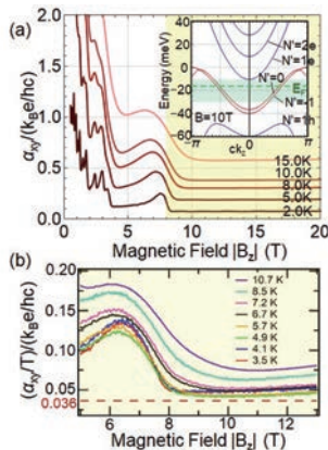
(a) グラファイトの量子極限におけるランダウ準位とトポジカル半金属的な量子化熱電ホール効果のモデル計算。(b) グラファイトの熱電ホール伝導度の実験結果。熱電ホールプラトーが観測された。
