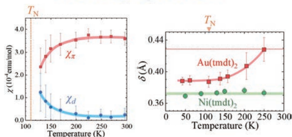
反強磁性金属 Au(tmdt) 2 (上) において核磁気共鳴測定 (左下) と放射線 X 線単結晶構造解析 (右下) の結果から、分子内電荷移動に伴って磁気相転移が生じることを見出した。
