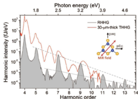
半導体 GaAs(011) に高強度中赤外光を集光して得られた高次高調波のスペクトル。赤線は透過配置でサンプル厚さ 30 μm の場合。黒線 (灰色塗りつぶし) は反射配置での場合。反射配置では非線形伝搬によるスペクトルの変化が少ないことを実験的に示した。
