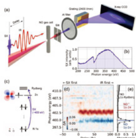
軟 X 線領域での一酸化窒素 (NO) 分子の過渡吸収スペクトル。(a) 実験配置。(b) ヘリウムガスで発生した軟 X 線パルスの典型的なスペクトル。(c) 軟 X 線吸収分光に対応する NO 分子のエネルギー準位。(d) 観測された過渡吸収スペクトル。(e) 軟 X 線レーザーで測定した定常状態での軟 X 線吸収スペクトル (黒丸) と、放射光で測定された軟 X 線吸収スペクトル (黒線)。
