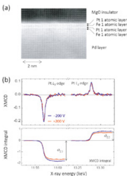
(a) 特徴的なナノ構造を有する新物質・材料薄膜の例。ありふれた材料の Fe・Pt・Pd等を原子レベルで積層し、新たな物性を示す薄膜デバイスを創成した。(b) オペランド X 線分光の例。外部から MgO 誘電層に電界をかけながらオペランド X 線分光を行い、界面 Pt 層の電子状態の変化を見出した。このような高品質薄膜デバイス研究と X 線分光研究の融合により、次世代不揮発性メモリの駆動技術として重要な電気磁気効果の物理機構を解明した。
