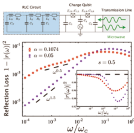
上図：サブオームミックス熱浴と結合した超伝導量子ビットを実現する超伝導回路。下図：マイクロ波の散乱ロスをマイクロ波の振動数の関数としてプロットしたもの。αは量子ビットと熱浴の結合定数。
