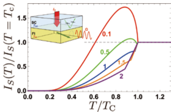
スピンプンピングによって生じる強磁性絶縁体から超伝導体へのスピン流の温度変化。挿入図：強磁性絶縁体 - 超伝導体接合の模式図。
