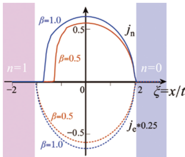
1次元ハバード模型の電流 j_c = e j_n とエネルギー流 j_e 。左右領域が電子密度 n = 1 および 0 の熱平衡状態から出発した後の時刻 t における空間分布。電子ホッピングを単位としてクーロン斥力 U = 8 、初期状態の逆温度 \beta = 0.5, 1.0 。 \xi \sim -2 付近に電流が消える領域が出現。
