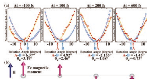
フェリ磁性 GdFeCo 合金の時間分解共鳴磁気光学カー効果の実験の結果。(a) 軟X線 FEL ( h\nu = 53 eV) でのエリソメトリ測定の実験データ (○) と三角関数でのフィッティング (実線)。赤と青のデータは互いに逆の磁場に対応している。(b) 実験結果から得られた外場 H に対する Fe の磁気モーメントの時間変化。フェムト秒の時間スケールでスピン反転が起きていることが分かる。
