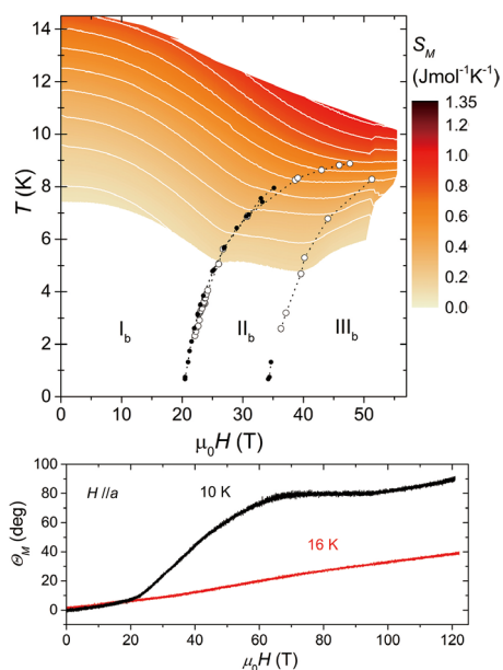
(a) AuGe フィルムを用いた測定された \text{BiCu}_2\text{PO}_6 の磁気熱量効果。(b) レーザー光を用いたファラデー回転角。磁気熱量効果の測定は等エントロピー変化 ( T(H) s) の測定と同意義であり、磁気相転移に伴う温度変化を観測している。ファラデー回転角はシングルターンコイルを用い 120 T まで測定しており、60 T 付近、90 T 付近で相転移を検出した。
