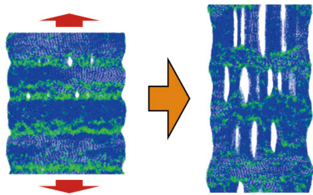
伸長下の結晶性高分子の破壊。アモルファス層に空孔が生成し、破けていく。
