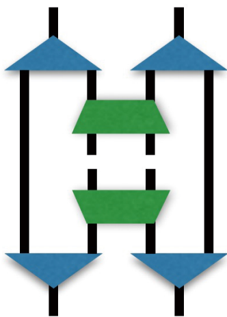
2 サイト演算子の繰り込み変換を定義する超演算子。多角形はテンソルを表し、Multi-scale entanglement renormalization ansatz (MERA) を用いて計算される。 A super-operator that defines renormalization transformation of two-site operators. Each tensor represented by a polygon is computed through MERA.
