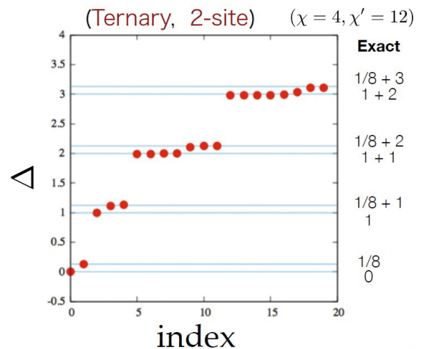
繰り込み超演算子の固有値問題から求められる2次元イジングモデルのスケールング次元。
