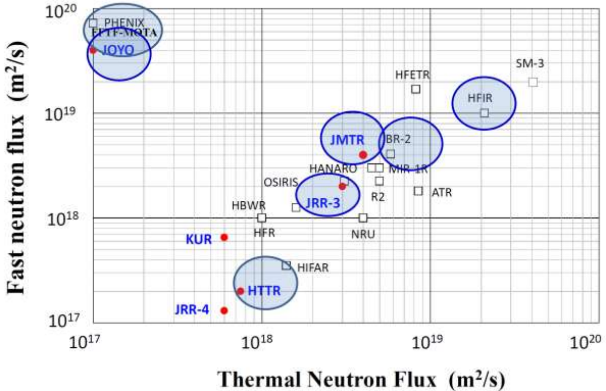
図 1-11 国内外の主な研究炉の比較 (参考文献[30])
