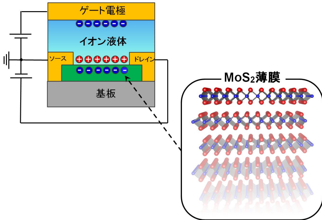
図1：二硫化モリブデン MoS 2 を用いた電気二重層トランジスタ構造
