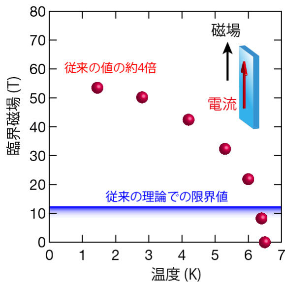
図2：MoS 2 -EDLT における面内磁場下における臨界磁場の温度依存性
