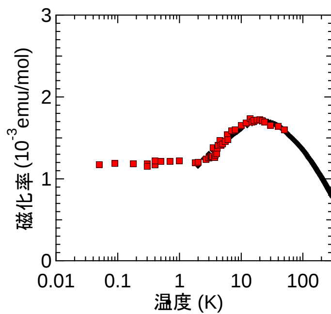
図3 発見した \kappa -H 3 (Cat-EDT-TTF) 2 の磁化率の温度依存性 約 3K (-270.15℃) から 50mK (-273.10℃) という極低温領域まで磁化率が一定となっており、 これは量子スピン液体状態を示していることがわかる。
