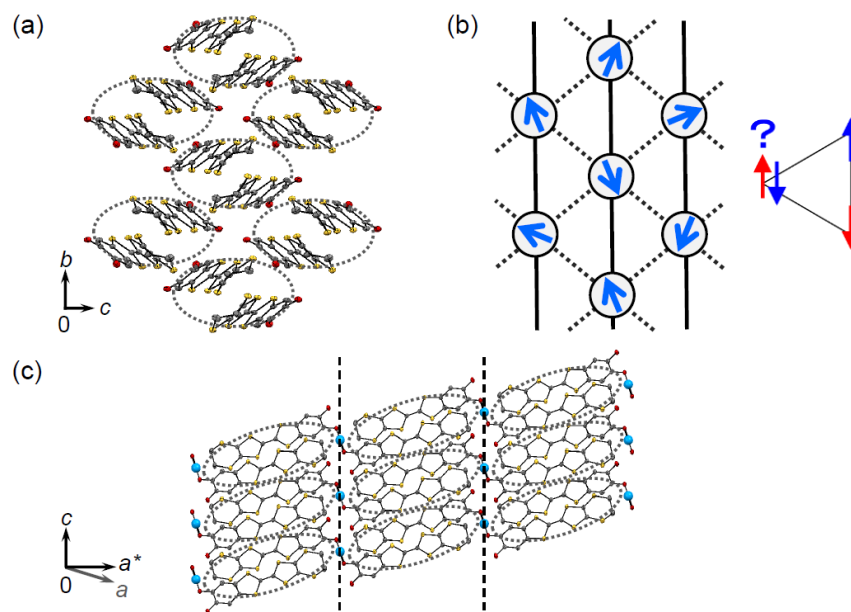
図1 発見した \kappa\text{-H}_3(\text{Cat-EDT-TTF})_2 の構造
