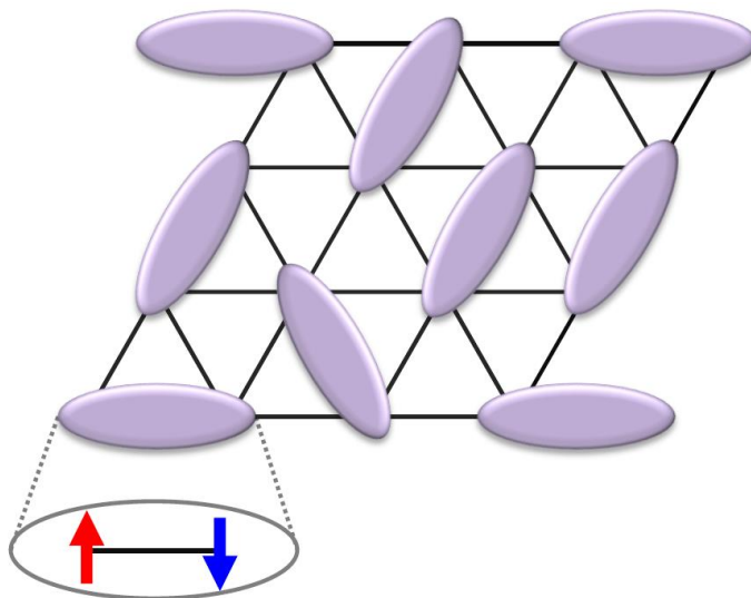
図2 P.W. Anderson 教授により提唱された RVB（共鳴原子価結合）状態の模式図
