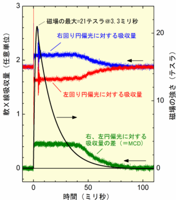
図2 CoFe/MnIr 薄膜の Co L_3 吸収端 (780 電子ボルト) における軟X線 MCD 測定結果。説明は本文参照。
