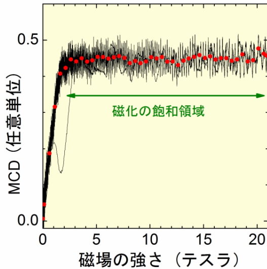
図3 図2のMCD測定結果から得たコバルト(Co)だけの磁化曲線。 黒線は測定データを直接プロットしたもので、赤丸は精度を上げるために0.25テスラごとに生データを平均化した値のプロット。
