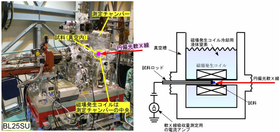
図1 パルス強磁場発生装置を備えた軟X線 MCD 測定装置（左）と、測定チャンバーの断面模式図（右）。
