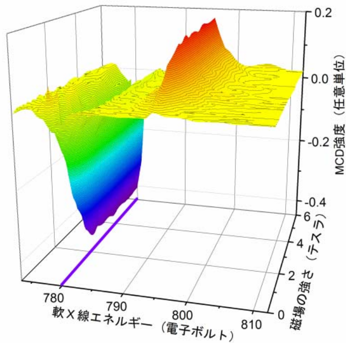
図4 図2と同様の測定を軟X線のエネルギーを変化させながら繰り返し行うことで得た軟X線MCDスペクトルの磁場依存性。
