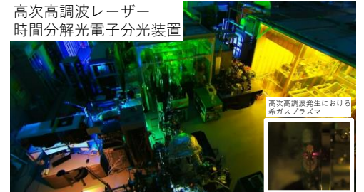
高次高調波レーザー 時間分解光電子分光装置
