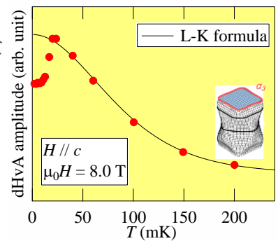
CeCoIn 5 の量子振動振幅の温度依存性 H. Shishido et al., Phys. Rev. Lett. (2018)
