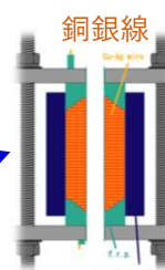
銅銀線 繊維強化プラスチック
